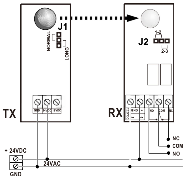
Figura 2. Collegamento con 24VDC o 24VAC
